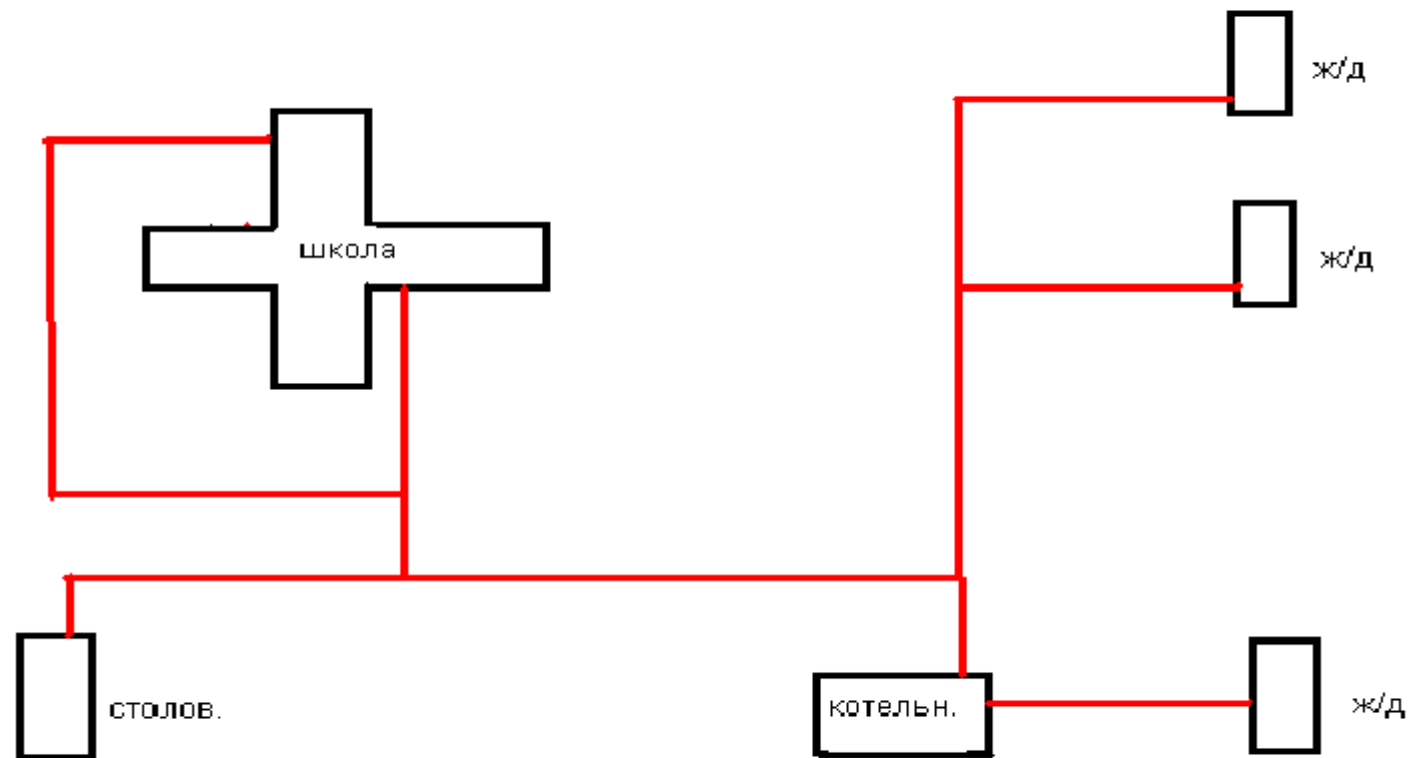
Схема тепловой сети с.Закопы
