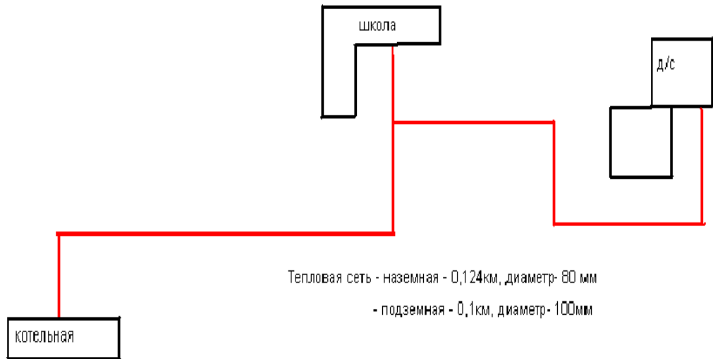
Схема тепловой сети с.Кадное
